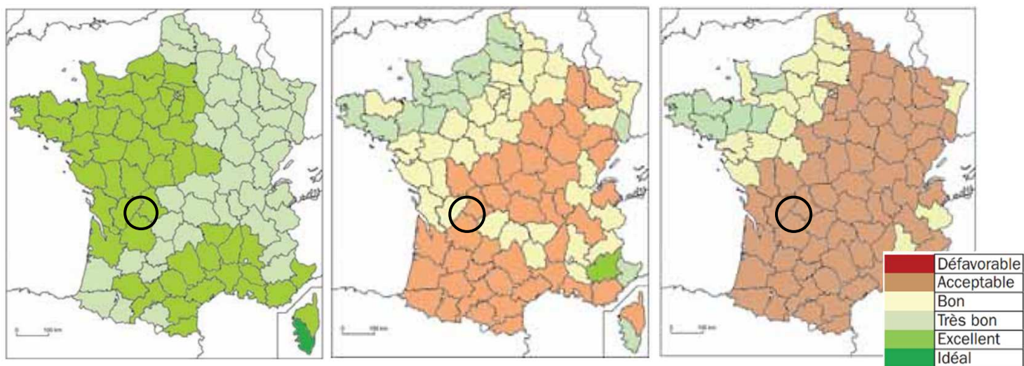
ICT des mois de juillet et août sur le période 1980-200 (gauche) 2080 (centre) et 2100 (droite)
