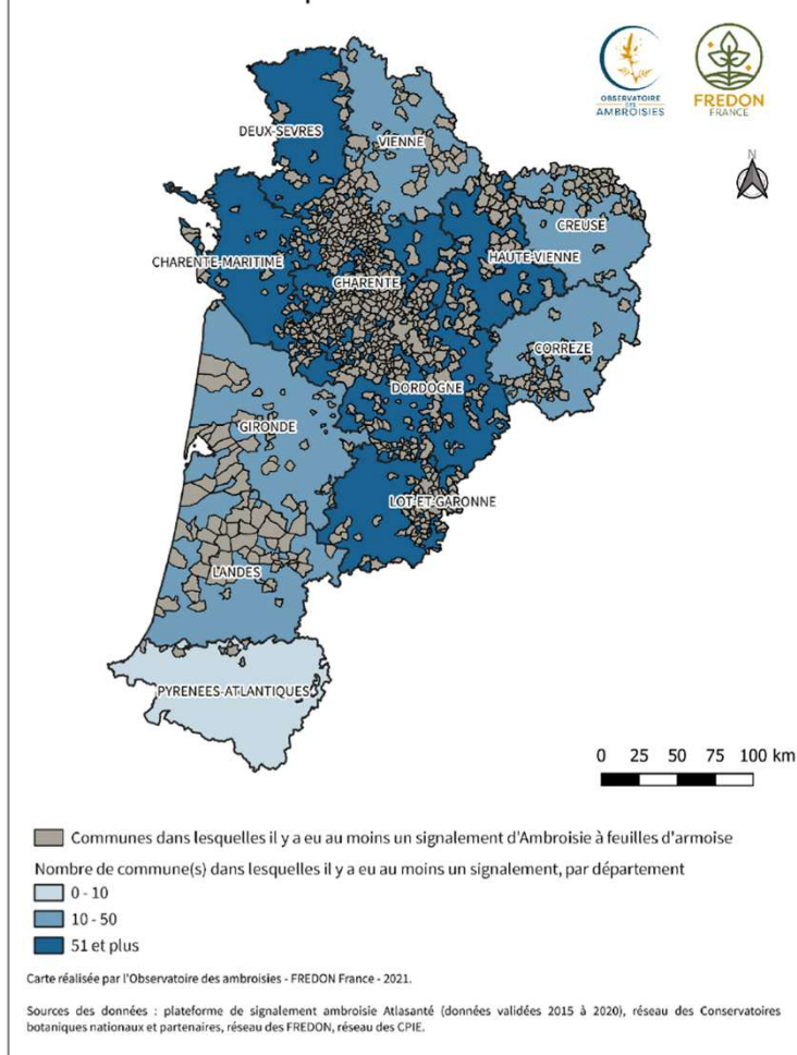
Etat des connaissances sur la répartition de l'Ambroisie à feuilles d'armoise ( Ambrosia artemisiifolia L.) en Nouvelle aquitaine entre 2001 et 2021
