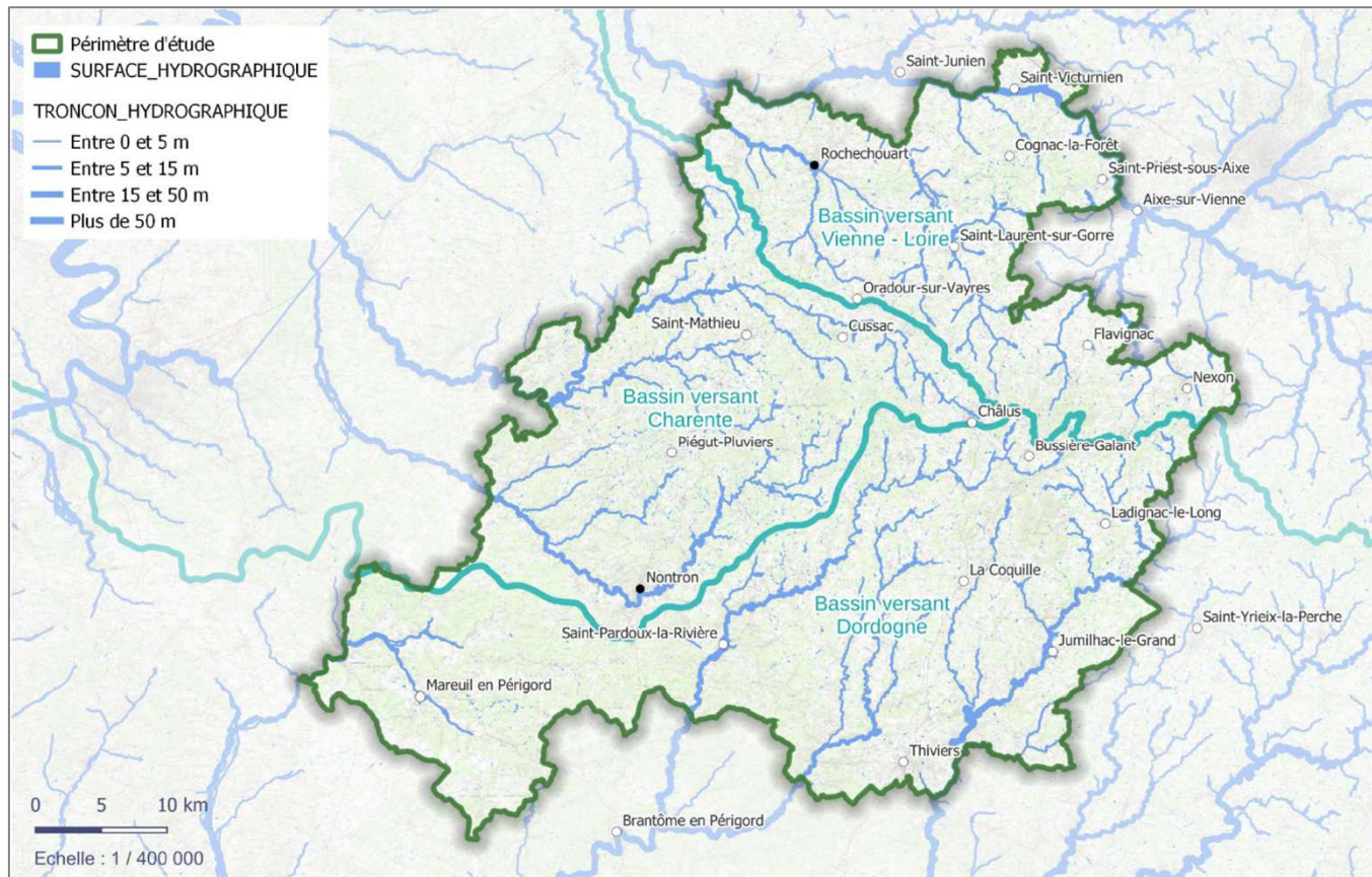
Réseau hydrographique du territoire du Parc Périgord-Limousin
