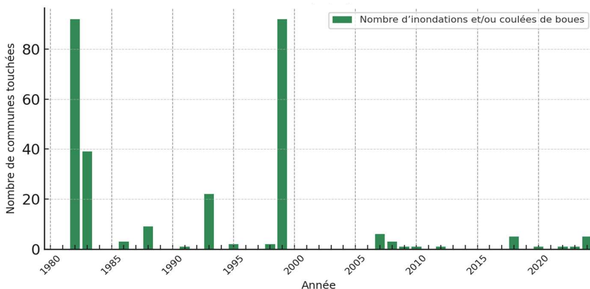
Evolution du nombre d'arrêtés CatNat inondations par année, (1982-2024), Parc PL. Données BDD Gaspar, septembre 2024
